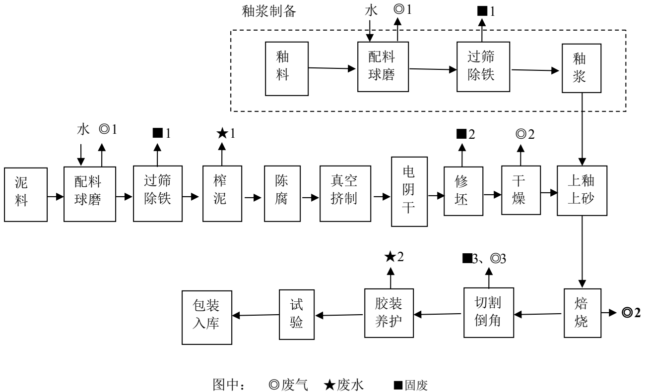
图 3-1 生产工艺流程及产污节点图
